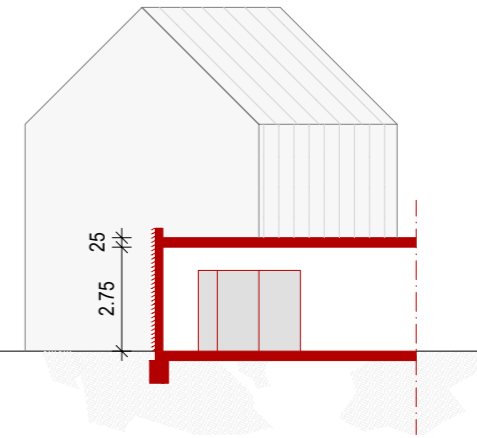
Schnitt B-B Arkaden M 1-200
