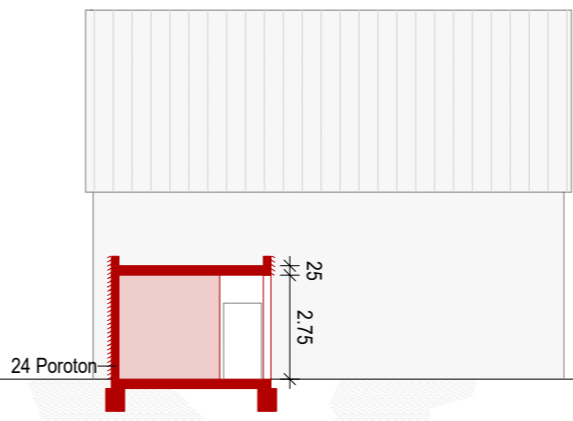
Schnitt A-A Arkaden M 1-200
