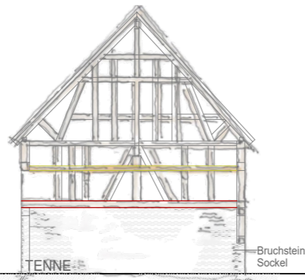
Schnitt A-A Scheune M 1-200
